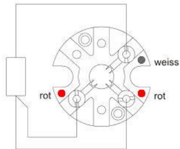
1xPt100 3-Leiter
