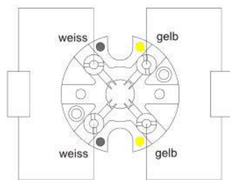
2xPt100 2-Leiter
