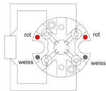
1xPt100 4-Leiter
