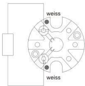
1xPt100 2-Leiter
