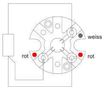
1xPt100 3-Leiter
